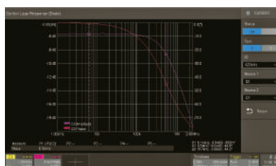
ボード線図
